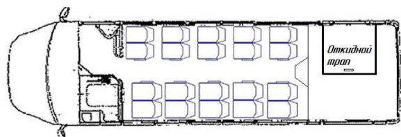
Автобус городской «Нижегородец» VSN-700
